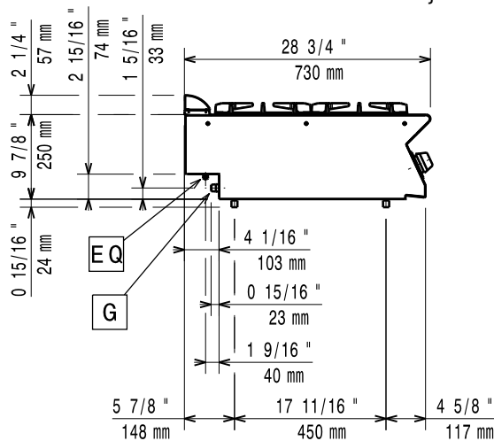
Zij aanzicht
